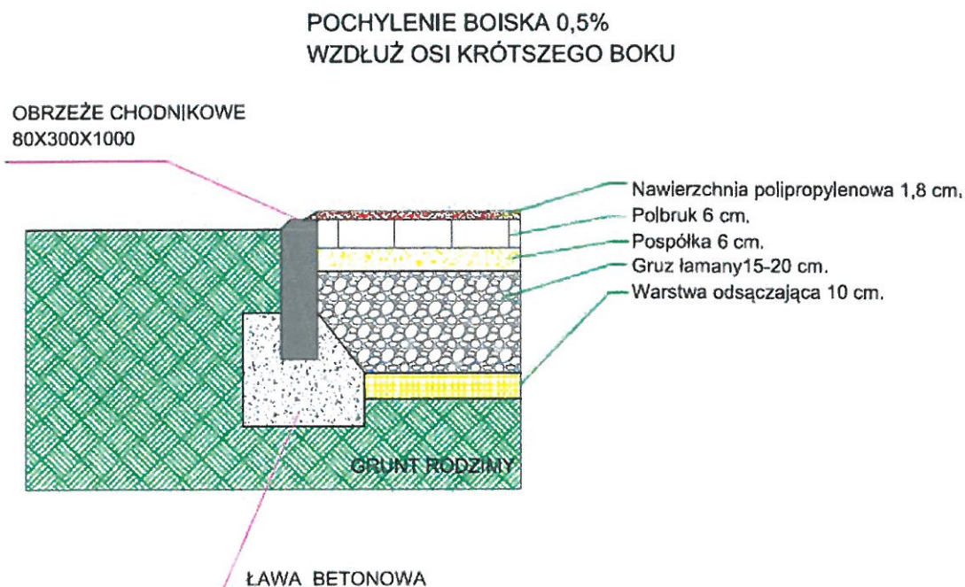
Rys. nr 1 Podbudowa pod nawierzchnię polipropylenową:
