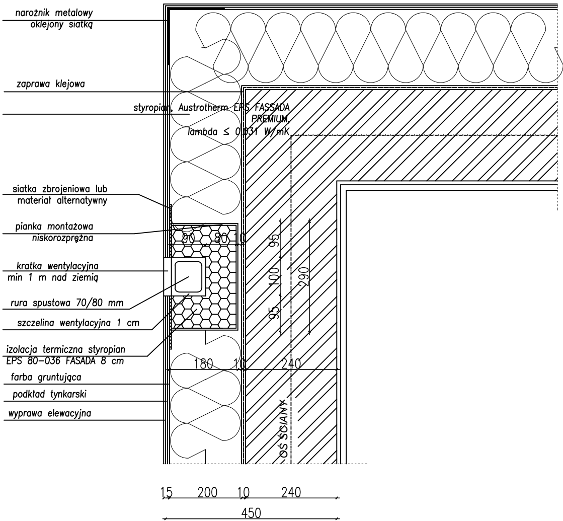
SZCZEGÓŁ OCIEPLENIA RURY SPUSTOWEJ
