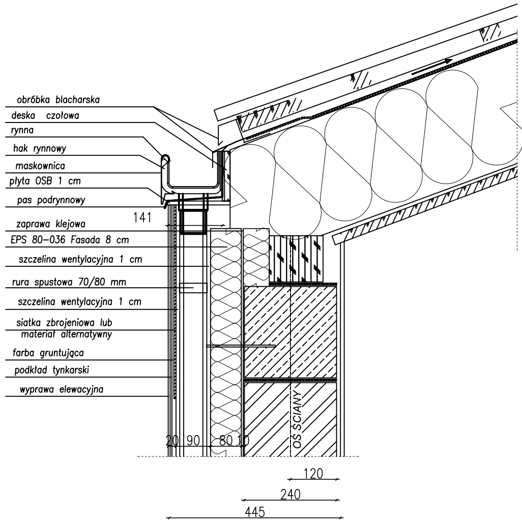
SZCZEGÓŁ POŁĄCZENIA RYNNY I RURY SPUSTOWEJ
