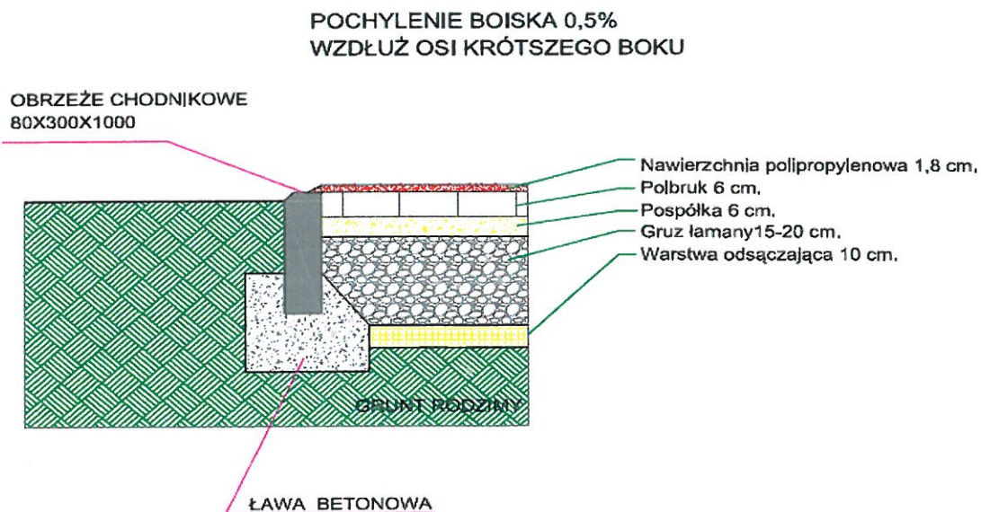
Rys. nr 1 Podbudowa pod nawierzchnię polipropylenową:
