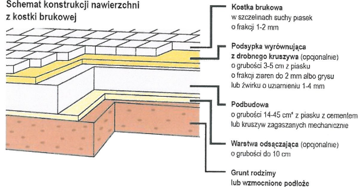
Schemat warstw nawierzchni placów
